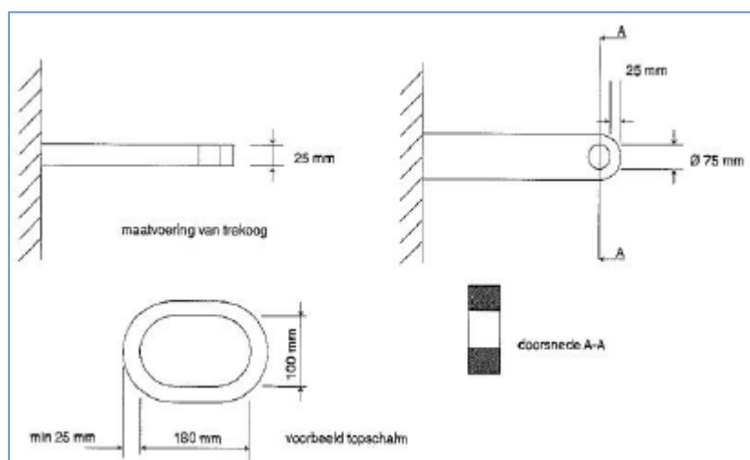
Figuur 2: Maatvoering trekoog en topschalm
